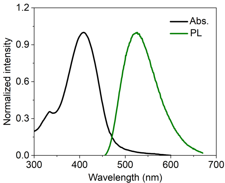
乙醇溶剂绿光量子点吸收光谱、光致荧光曲线图
