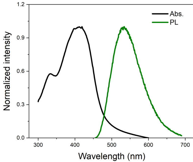
水溶剂绿光量子点吸收光谱、光致荧光曲线图
